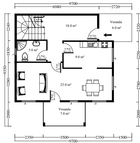
ZEMİN KAT 70 m 2
