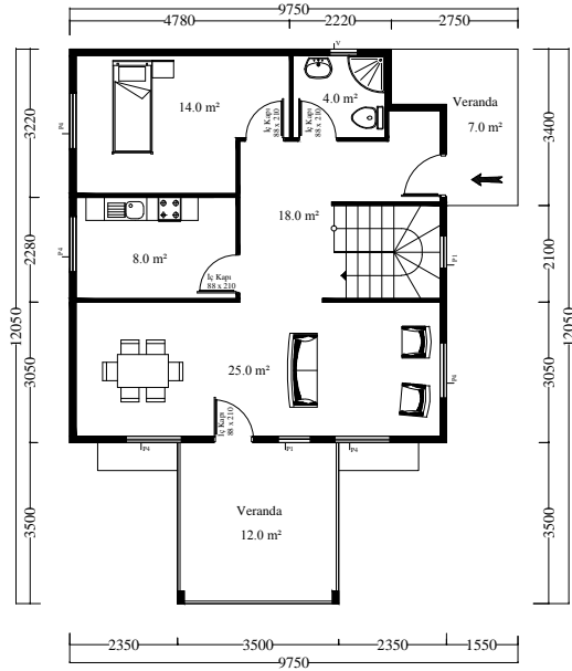
ZEMİN KAT 88 m 2
